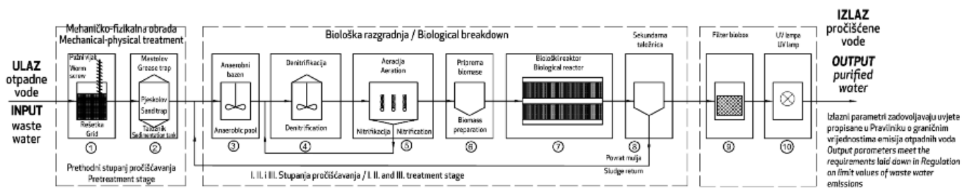
Tehnološka shema rada:
