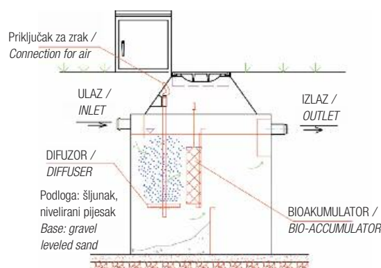
UGRADNJA BIOJAME / INSTALACION
