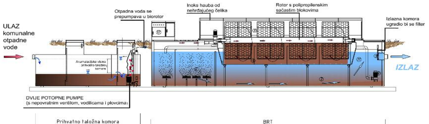
Tehnološka shema rada:
