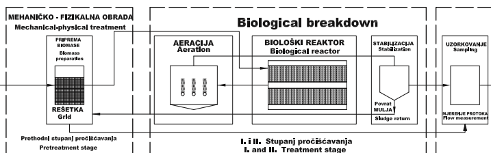
Schema rada biorotora kapaciteta do 600 ES / Operation schematic of 600 PE biorotor
